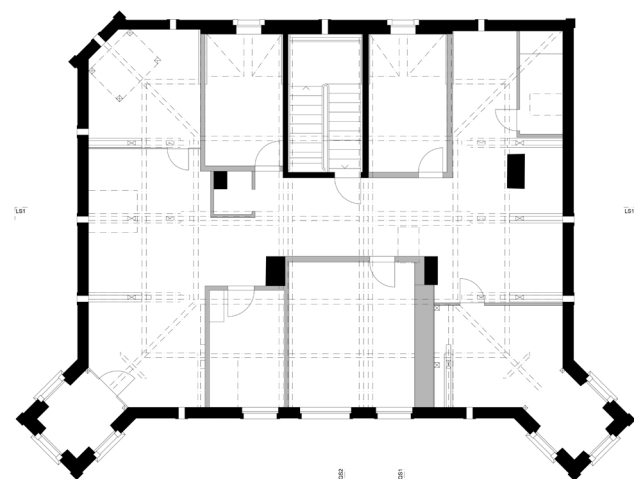
Grundriss Dachgeschoss
